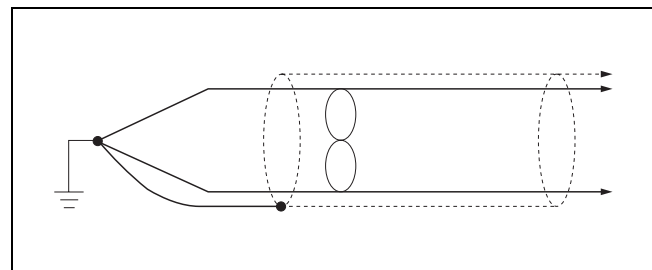
Bild 6 Abgeschirmtes Thermoelement mit geerdeter Lötstelle. Verdrillte Ausgleichsleitung
