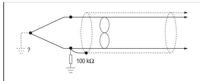
Bild 8 Thermoelement mit zweifelhafter Erdung. Verdrillte, abgeschirmte Ausgleichsleitung
