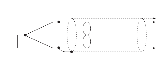
Bild 7 Thermoelement mit geerdeter Lötstelle. Abgeschirmte Ausgleichsleitung
