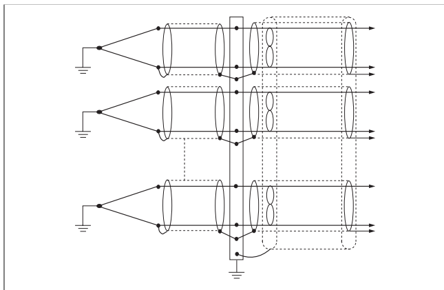
Bild 10 Einzel verdrehte, abgeschirmte Ausgleichsleitungen im Anschluß an vieladrige Ausgleichsleitungen mit einzeln verdrehten Leiterpaaren Abschirmung um Einzelpaare und Kabel
