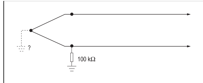
Bild 5 Thermoelement mit zweifelhafter Erdung Unverdrillte, ungeschirmte Ausgleichsleitung
