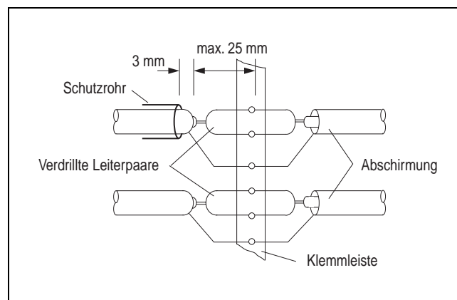
Bild 12 Die Verbindung von Abschirmungen an Klemmleisten. Das Schutzrohr muß bis 3 mm vor das Ende der Abschirmung reichen. Freiliegende Abschirmungen müssen mit Klebeband geschützt werden.
