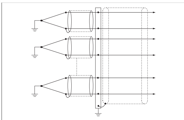
Bild 11 Einzel verdrehte, abgeschirmte Ausgleichsleitungen an vieladrigem Kabel mit äußerer Abschirmung
