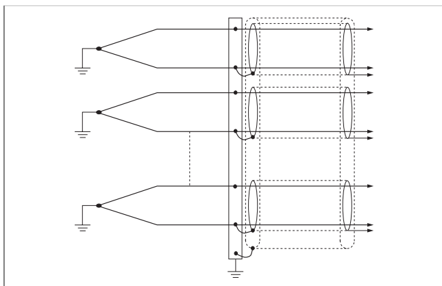
Bild 9 Einzelne, unabgeschirmte Thermoelemente und Ausgleichsleitungen an vieladrige, paarweise verdrehte Ausgleichsleitungen mit Einzel- und Gesamtabschirmung angeschlossen
