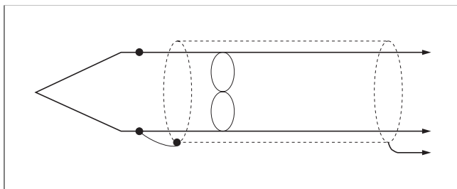
Bild 4 Ungeerdetes Thermoelement Verdrillte, abgeschirmte Ausgleichsleitung
